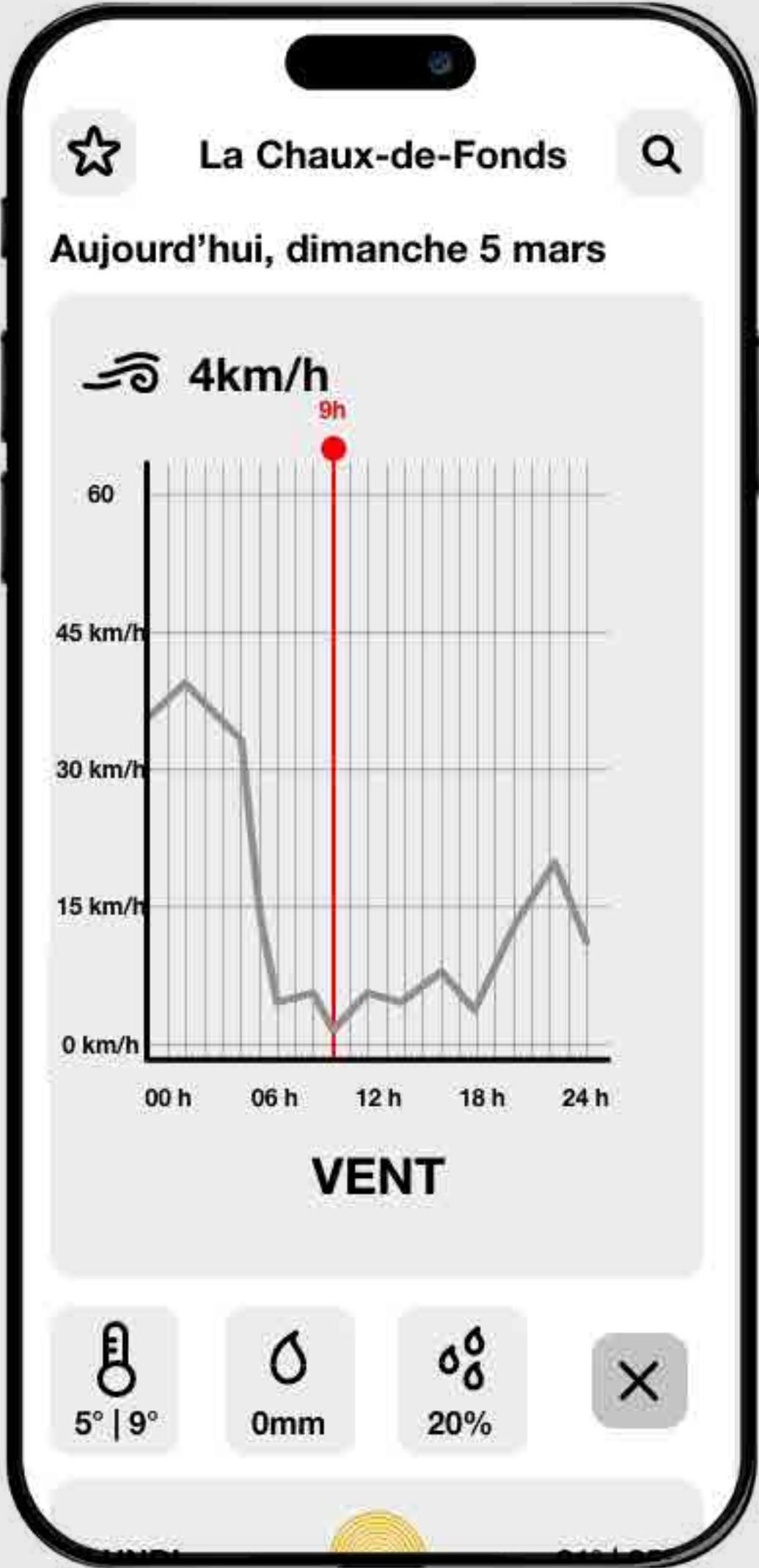
TENDANCE QUOTIDIENNE DU VENT
