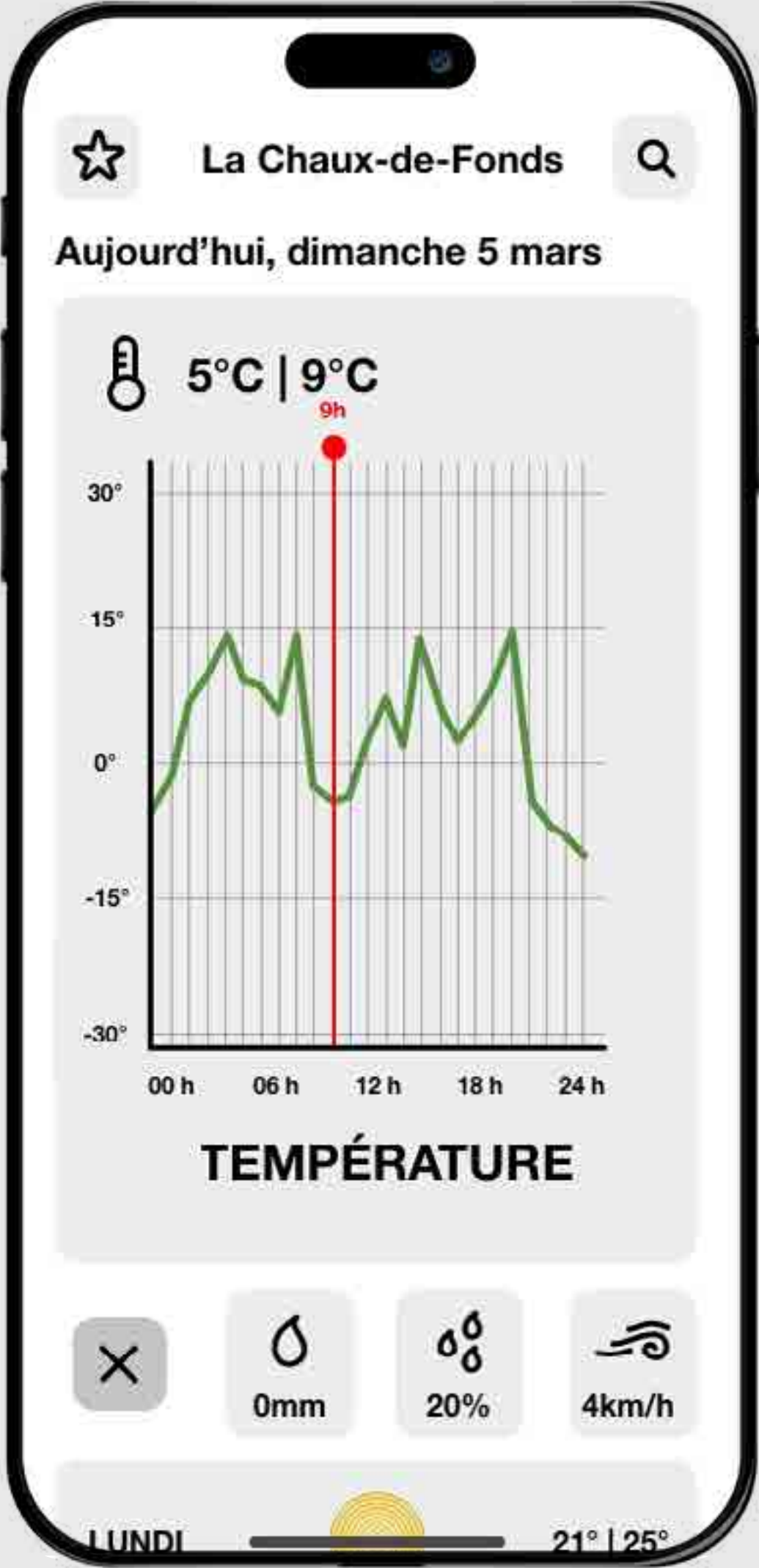
TENDANCE QUOTIDIENNE DE LA TEMPÉRATURE
