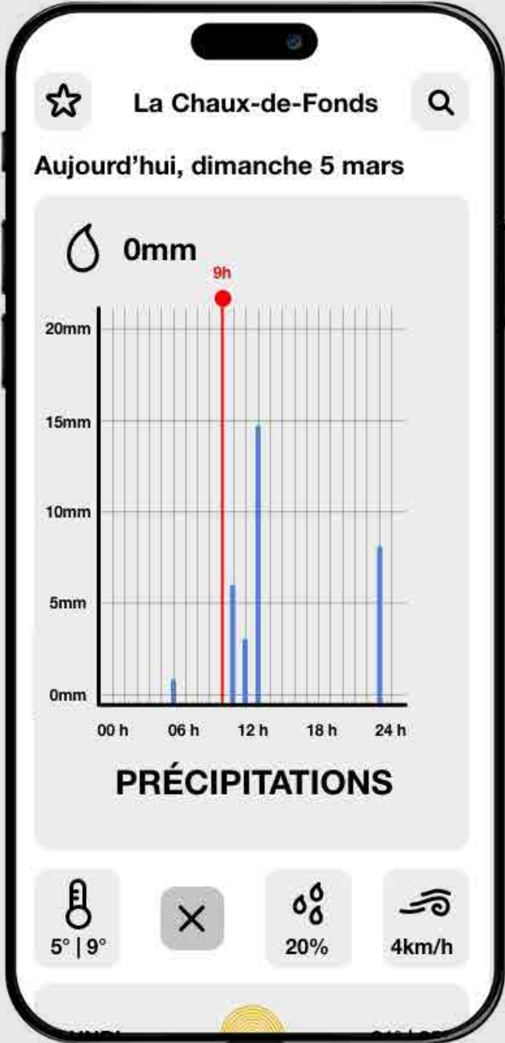
TENDANCE QUOTIDIENNE DES PRÉCIPITATIONS
