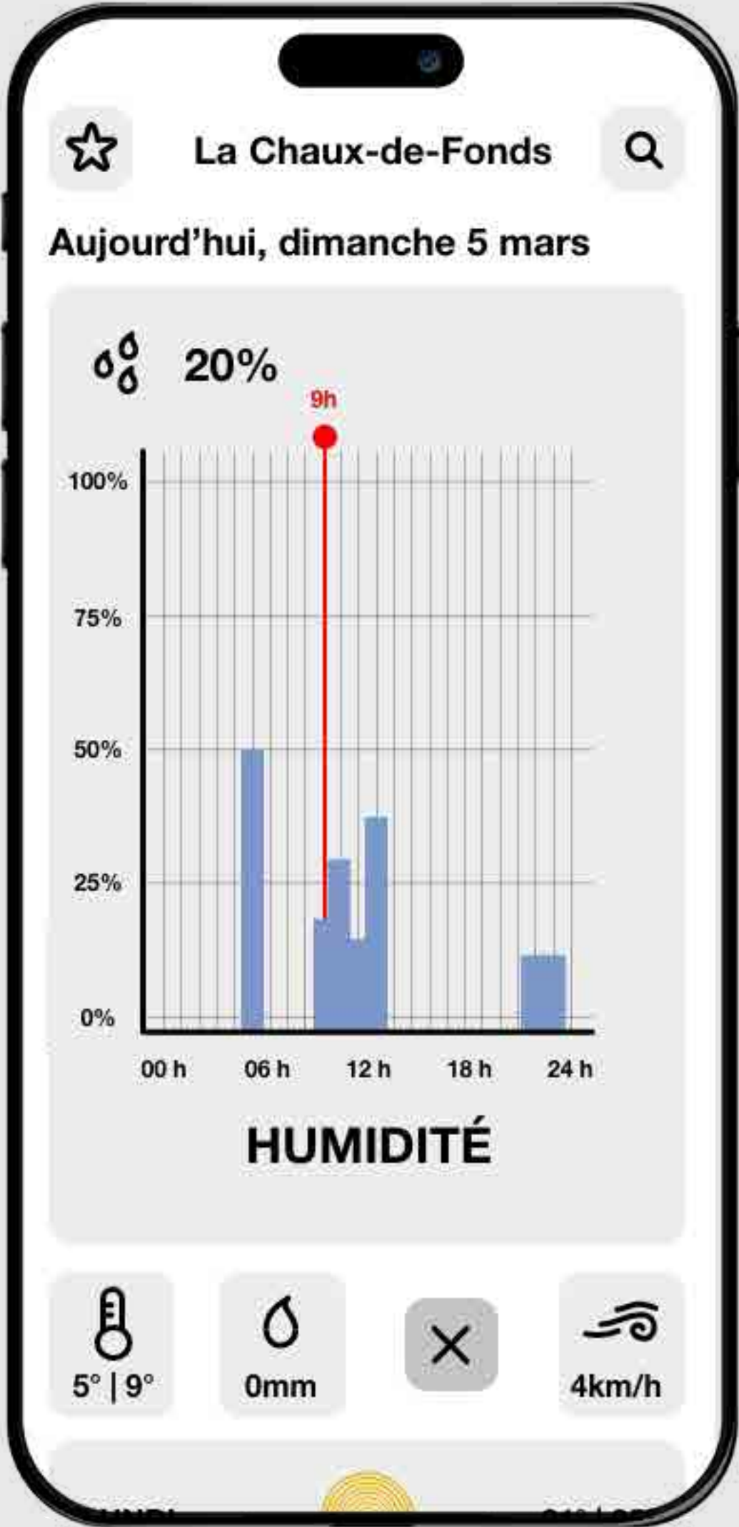
TENDANCE QUOTIDIENNE DE L'HUMIDITÉ
